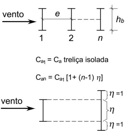
4 – Fator de proteção \eta para dois ou mais reticulados igualmente afastados
