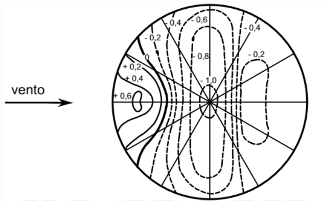
b) Vista superior – Linhas isobáricas dos coeficientes de pressão externa para f/d = 1/2
