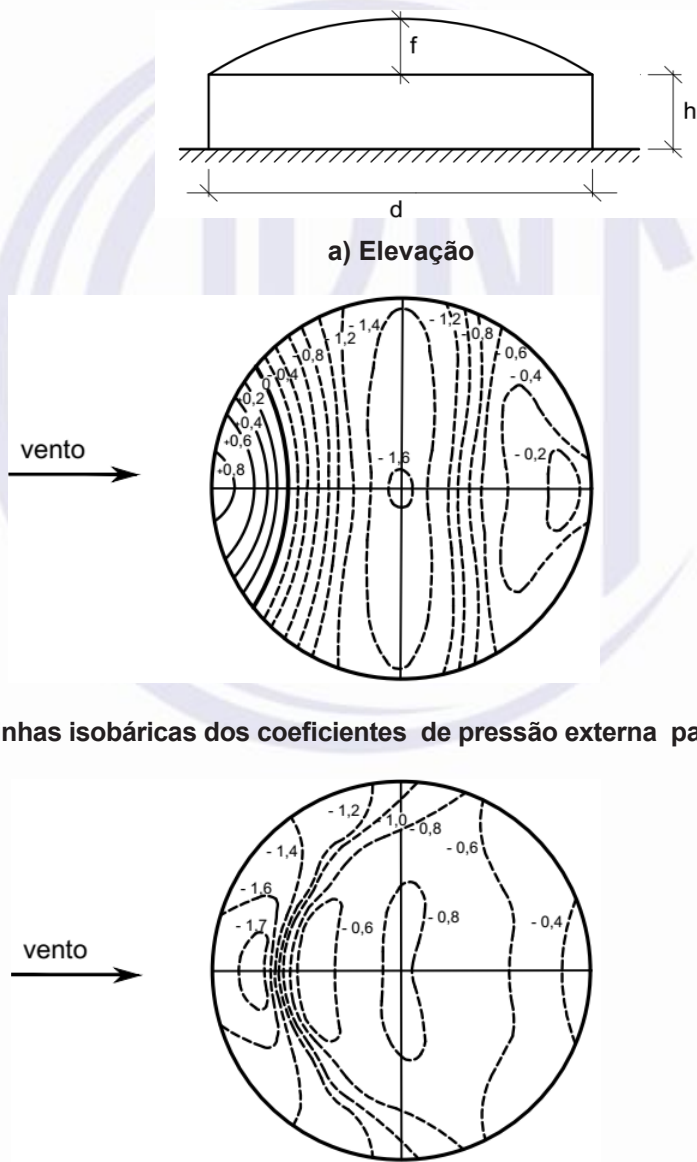
c) Vista superior - Linhas isobáricas dos coeficientes de pressão externa para f/d = 1/10 e h/d = 1
